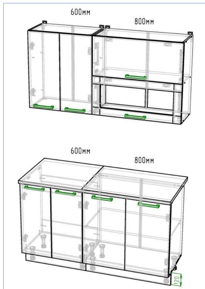
Регулировка петель:
