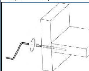
Сборка на конфирматы
